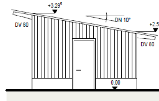
ANSICHT OSTEN
