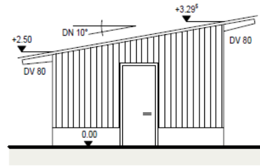
ANSICHT WESTEN
